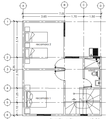
Proyecto ejecutivo de casa habitación (prototipo) para la empresa MG SISTEMAS a desarrollarse en el Estado de Tabasco.
