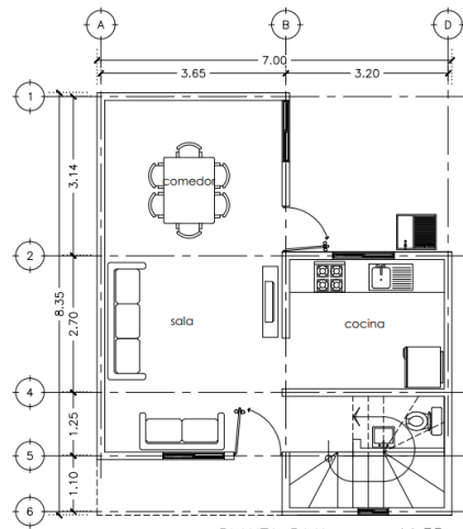
Proyecto ejecutivo de casa habitación (prototipo) para la empresa MG SISTEMAS a desarrollarse en el Estado de Tabasco.
