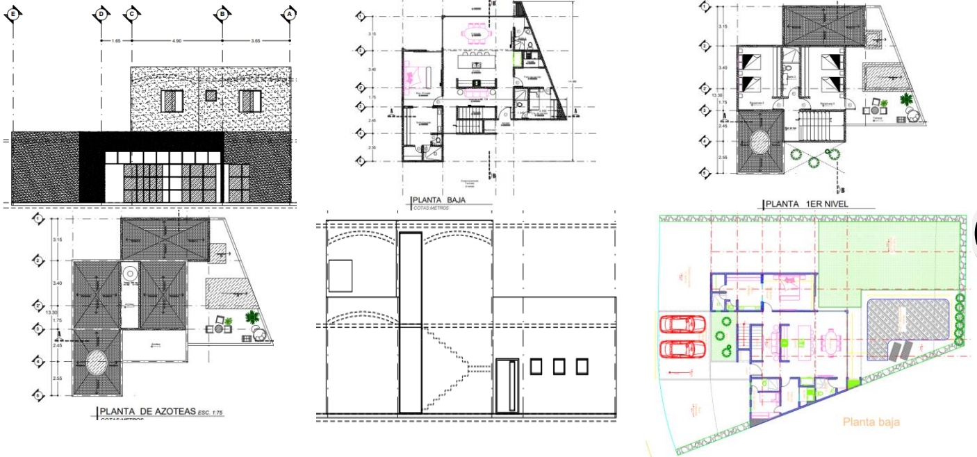
Proyecto ejecutivo de casa habitación a desarrollarse en Xolostoc, Morelos.
