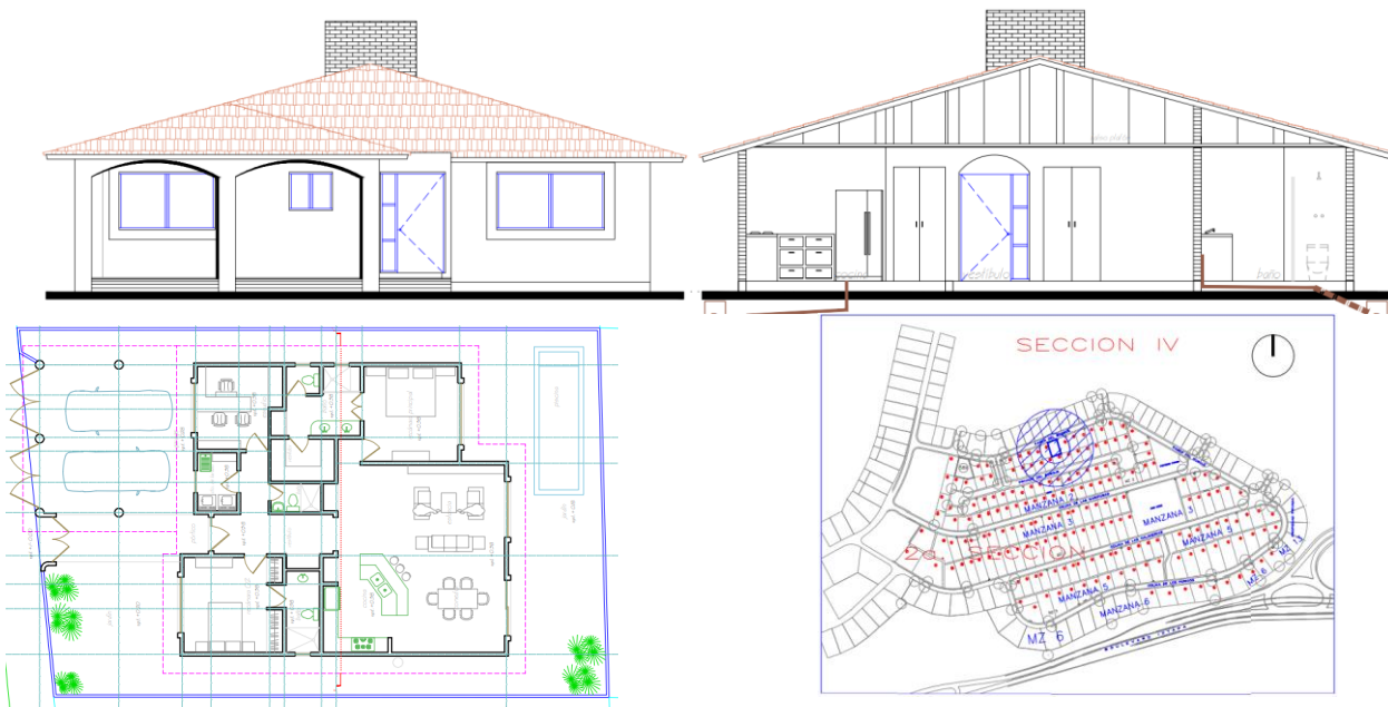
Proyecto ejecutivo de casa habitación ubicada en Ixtapa, Guerrero.
